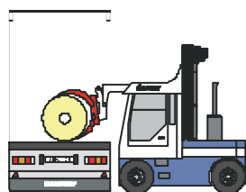
Liggande rulle mitt på bilen
