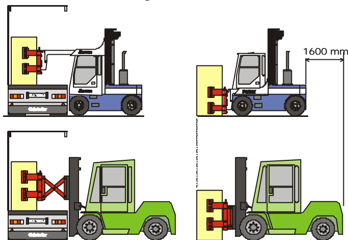
Ex. hantering av 5-tons rullar
